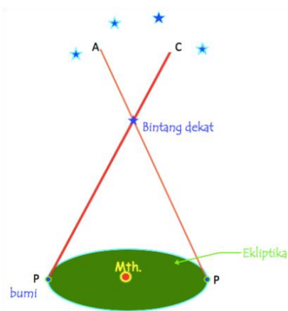
Gambar 3. Paralaks Bintang
