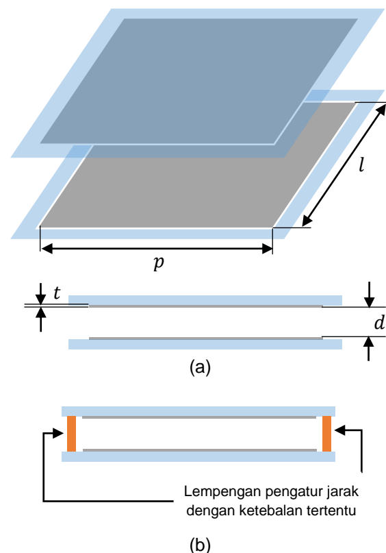
Gambar 2. (a) Rancangan elektroda plat
