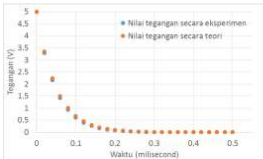
Gambar 10. Kurva perubahan tegangan V_c(t) (kapasitor elektroda plat sejajar berdielektrik udara dengan jarak antar elektroda 2 mm dan resistor 125 megaOhm)
